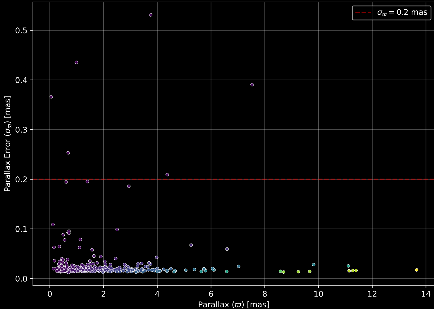
GALAH DR4 Field: [6775] Parallax Quality (n= 432)
