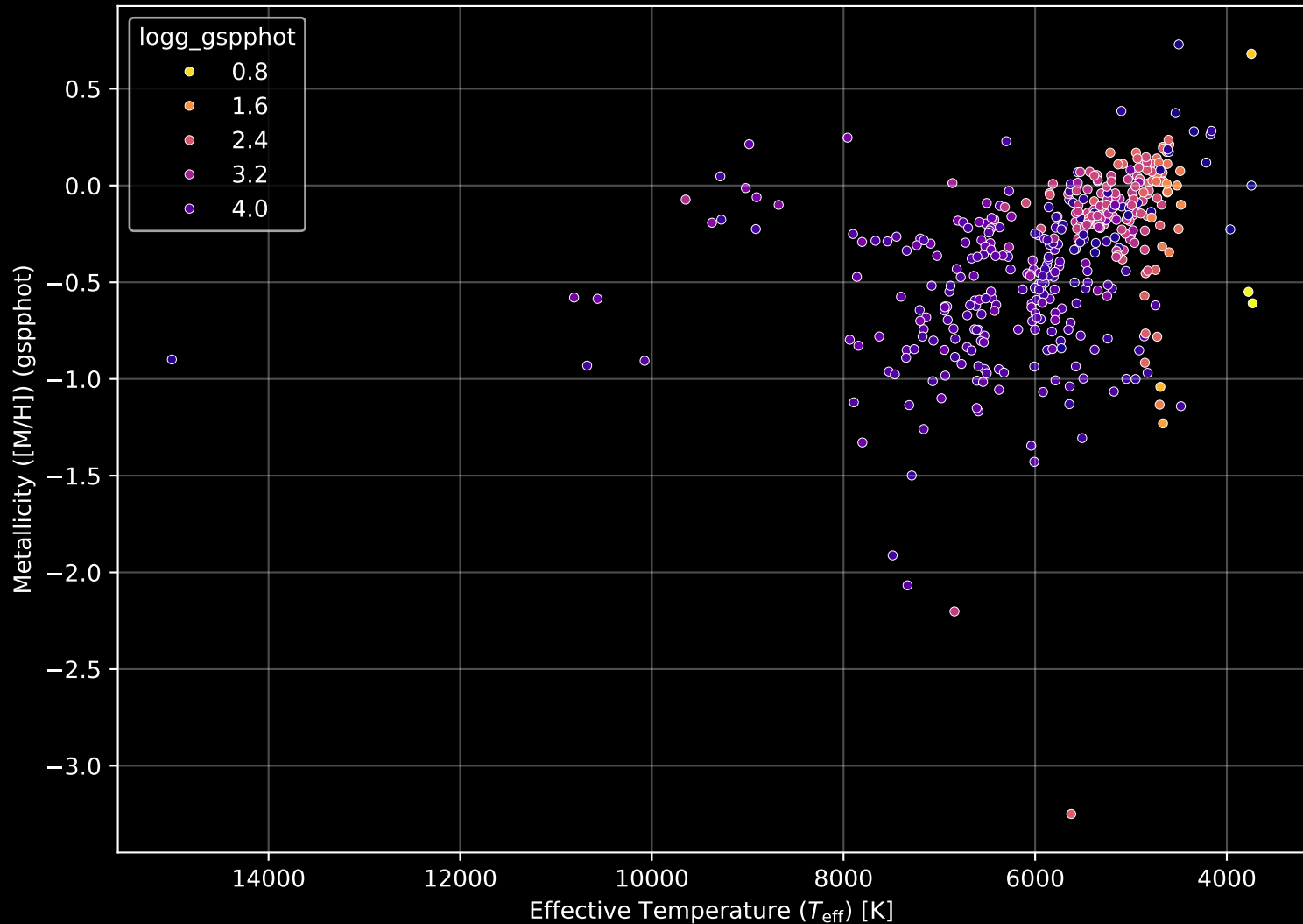
GALAH DR4 Field: [6775] Stellar Population Parameters (n= 432)
