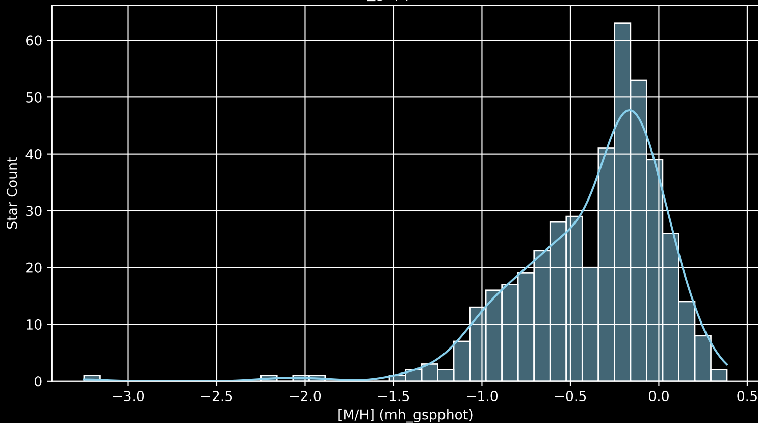
GALAH DR4 Field: [6775] [M/H] (mh_gspphot) (n= 430)
